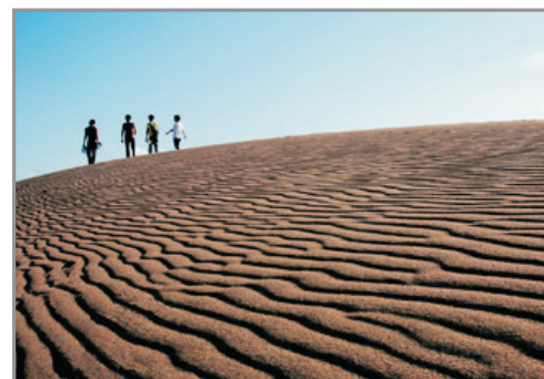
鳥取砂丘
